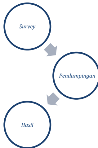
Gambar 1. Teknik Implementasi
