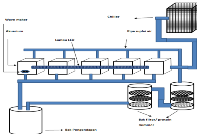
Gambar 1. Skema Penerapan Resirkulasi Akuarium Modular
